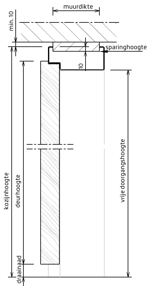
Verticale doorsnede
